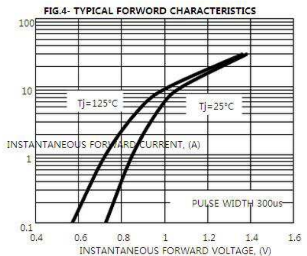
图4. 电性正向特性曲线
