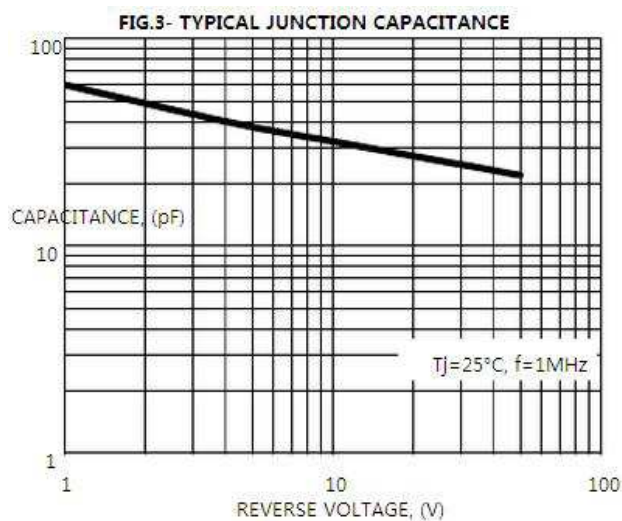
图3. 结电容随反向电压变化曲线
