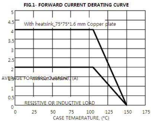
图1. 正向电流随温度变化曲线
