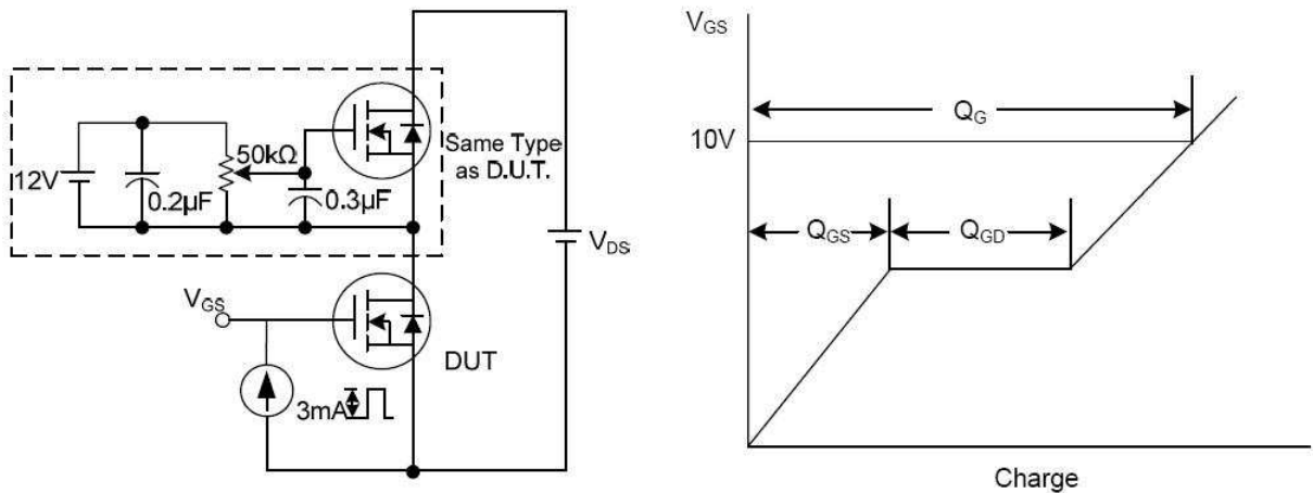
图12. 栅电荷测试
